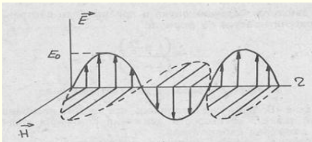
Рис.3. График световой волны ( http://studopedia.ru/1_89529_svet-kak-elektromagnitnaya-volna.html )
