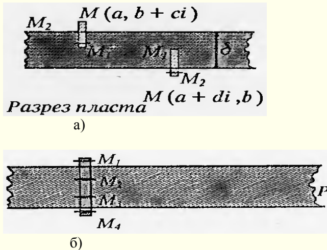
Рис.1. Физическая плоскость с точками на действительной и мнимой стороне [19]: а – чертёж 22, б – чертёж 27.
