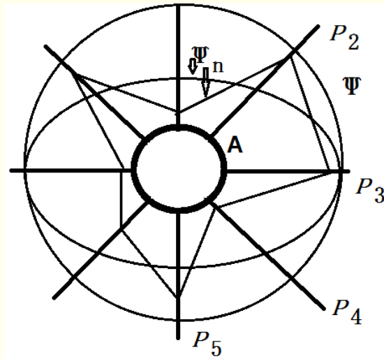
Рис.2. Физическая форма квантового явления. Условно показаны только пять плоскостей П.П. Флоренского: плоскость чертежа и P_2, P_3, P_4, P_5 , – плоскости, перпендикулярные чертежу, они же (след пересечения) – проективные линии в плоскости чертежа; А – Абсолют (мнимый диск на действительной стороне плоскости – лицевая сторона чертежа, диапир мнимой поверхности, находящейся на оборотной стороне чертежа), Ψ – совокупность вероятностей (состояние системы)
