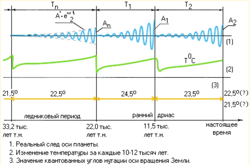
Рис. 5. «Изменение угла нутации – результат разницы скоростей нагревания (охлаждения) мелководной Арктики и глубоководной Антарктики. Период накопления энергии T_n > \dots > T_2 > T_1 Амплитуда колебания оси A_1 > A_2 > \dots > A_n », [4]
