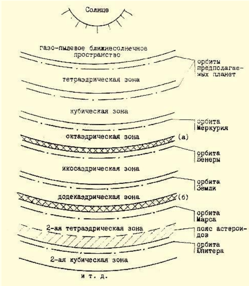
Рис. 1. Предполагаемое структурирование околосолнечного пространства
