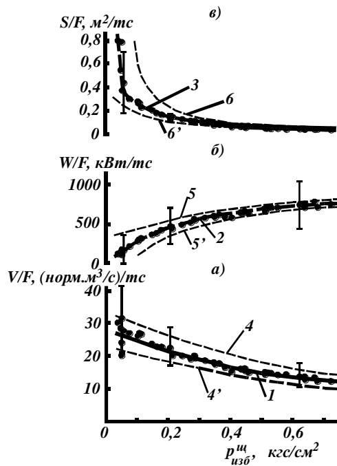
Рис.9. Основные характеристики плоского одноструйного сопла H = 102 мкм L = 0,8 мм, отнесенные к тяге в 1 тс, в зависимости от избыточного давления на входе в сопло: а) расход; б) теоретическая работа изотермического сжатия воздуха; в) несущая поверхность (совокупное поперечное сечение струй воздуха); 1,2,3 – кривые, полученные по методу наименьших квадратов; 4,4',5,5',6,6' – доверительные пределы при двусторонней доверительной вероятности 0,98
