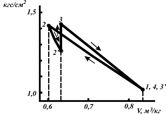
Рис.19. p^{эфф} - V диаграмма бестопливного монотермического двигателя при изотермическом сжатии в компрессоре.
