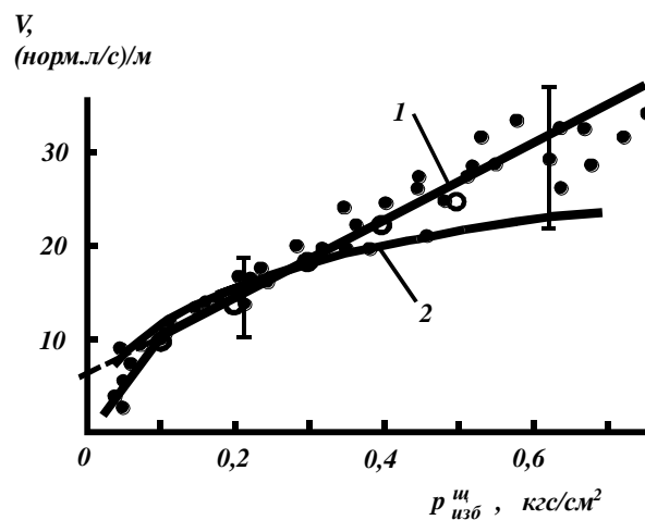
Рис.7. Расход воздуха в плоском одноструйном сопле H = 102 мкм L = 0,8 мм в зависимости от избыточного давления на входе в сопло: 1 – измерения автора; 2 - расчет по формуле ( 32 ); \circ - измерения сотрудников НПО им.С.А.Лавочкина
