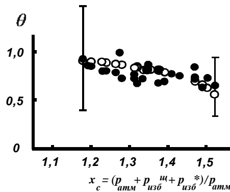
Рис.15. Зависимости величин \theta , определенных экспериментальным и теоретическим путем, от суммарной степени сжатия x_c : ● - эксперимент; ○ - расчет
