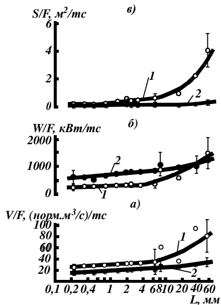
Рис.11. Основные характеристики плоского одноструйного сопла H = 102 мкм, отнесенные к тяге в 1 тс, в зависимости от длины щели: а) расход; б) теоретическая работа изотермического сжатия воздуха; в) несущая поверхность (совокупное поперечное сечение струй воздуха); 1 - при избыточном давлении воздуха на входе в щель 0,1 кгс/см 2 ; 2 - при 0,4 кгс/см 2
