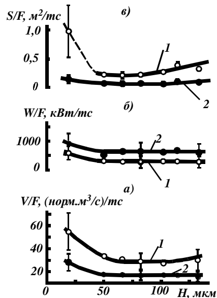
Рис.10. Основные характеристики плоского одноструйного сопла L = 0,8 \text{ мм} , отнесенные к тяге в 1 \text{ тс} , в зависимости от зазора щели: а) расход; б) теоретическая работа изотермического сжатия воздуха; в) несущая поверхность (совокупное поперечное сечение струй воздуха); 1 - при избыточном давлении воздуха на входе в щель 0,1 \text{ кгс/см}^2 ; 2 - при 0,4 \text{ кгс/см}^2
